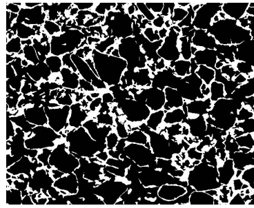
Fig. 4. Somme des argiles, pores, cracks et limites de grains détectés par l'algorithme à la première étape
