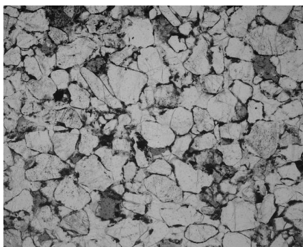
Fig. 1. Image initiale du grès de Tumlin (100 \times , lumière naturelle)
